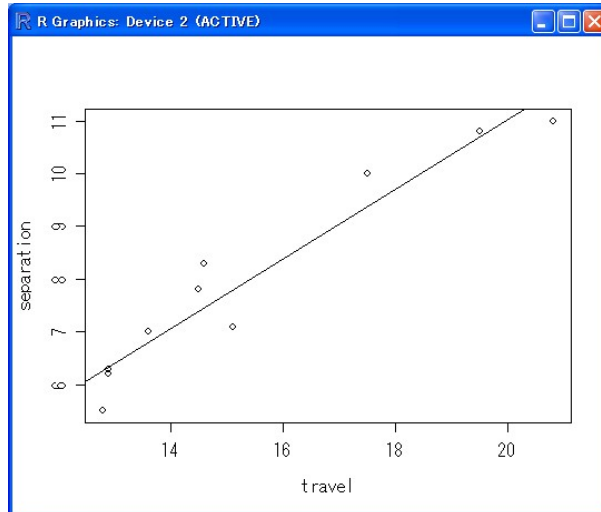
図 2.7: 回帰直線
